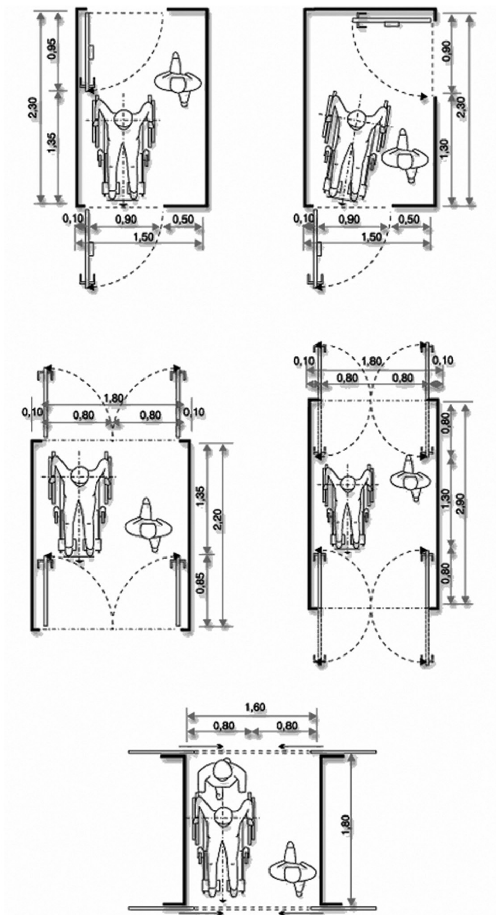
Σχεδιασμός προσβάσιμων ανεμοφρακτών εισόδου
